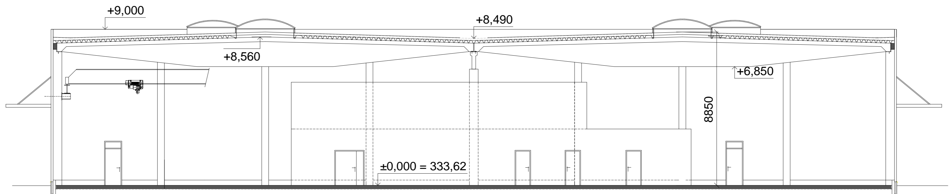
ŘEZ A - A - CUT A - A
